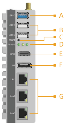
正视图接口
